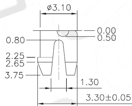
DETAIL Y
