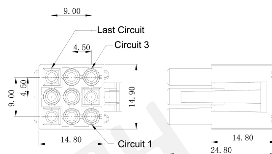
MR-C4500HF-3*03P
