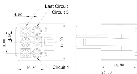
MR-C4500HF-2*03P
