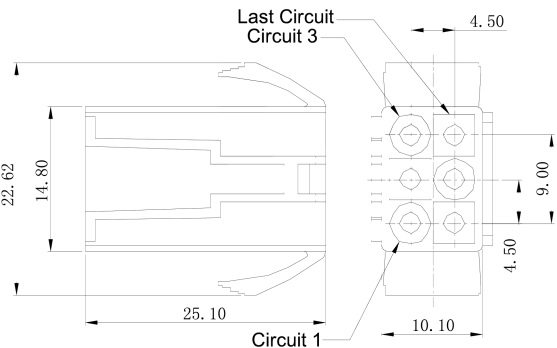
MR-C4500HM-2*03P
