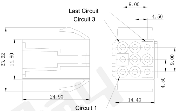
MR-C4500HM-3*03P
