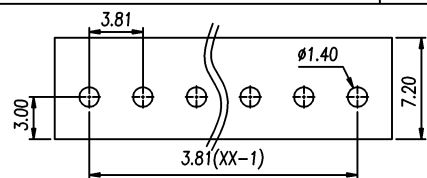
P.C.B. LAYOUT
