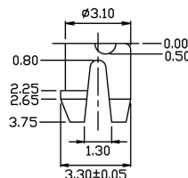
DETAIL Y
